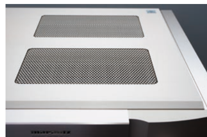
5mm铝质机箱散热盖板，既可以散热，又能屏蔽外来电磁干扰的作用，更减少分布电感之功效
